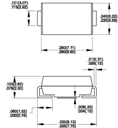
DO-214AB (SMC)
