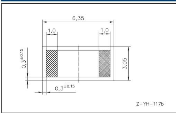
Layout Typ B / Layout type B
