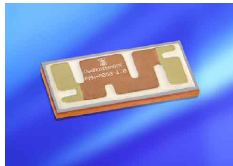
Bauform/Size 2512
