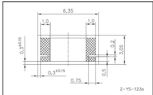
Layout Typ C / Layout type C
