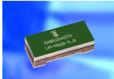
Bauform/Size 0805
