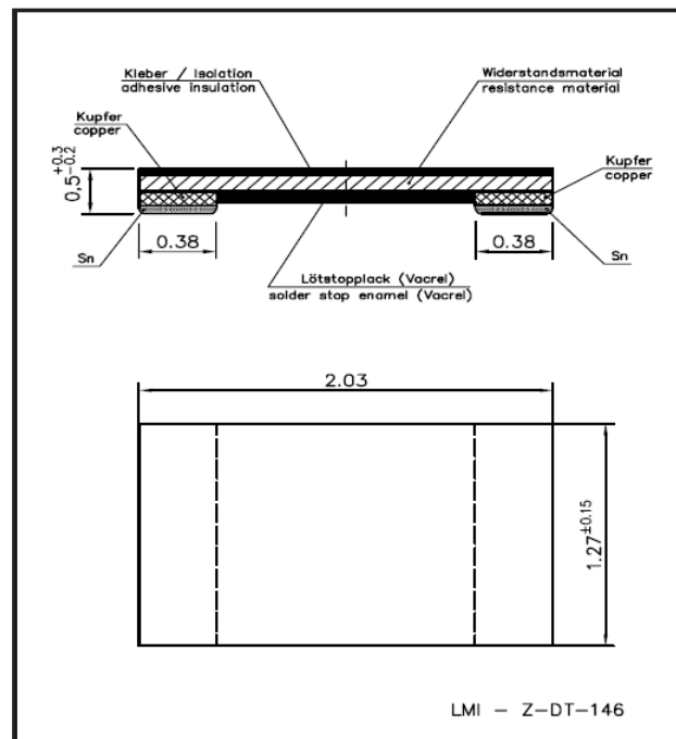
Bauform/Size 0805
