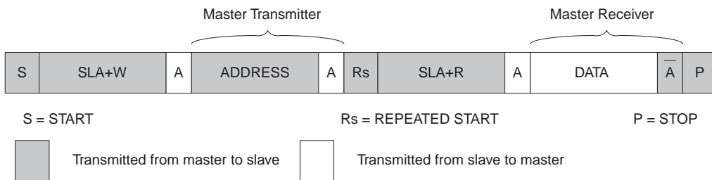
Figure 97. 几种 TWI 模式联合访问串行 EEPROM
