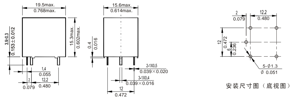
外形尺寸图
