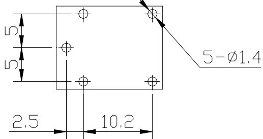
安装图
