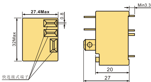
外形图
