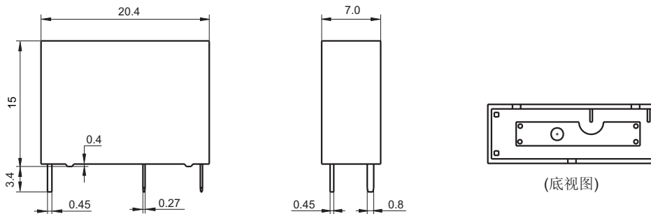
外形图
