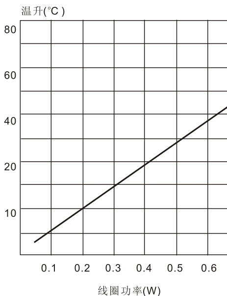
线圈温升
