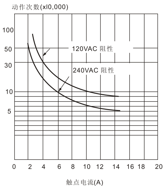
寿命曲线
