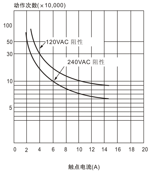
寿命曲线
