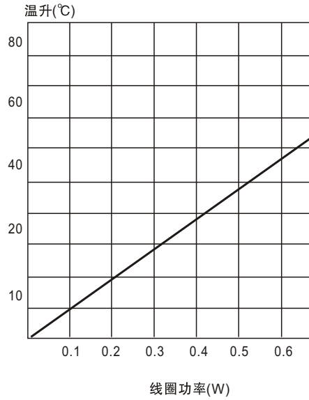
线圈温升
