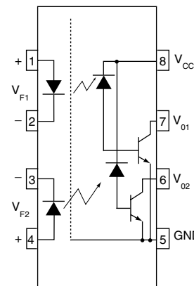
HCPL-2530/HCPL-2531
