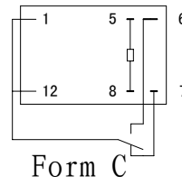
接线图
