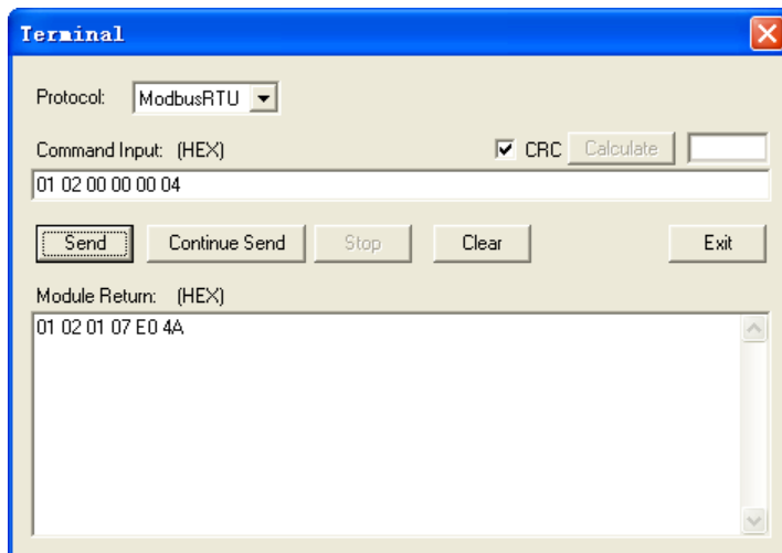
图2.2.6.c (ModbusRTU协议时的命令与返回信息)
