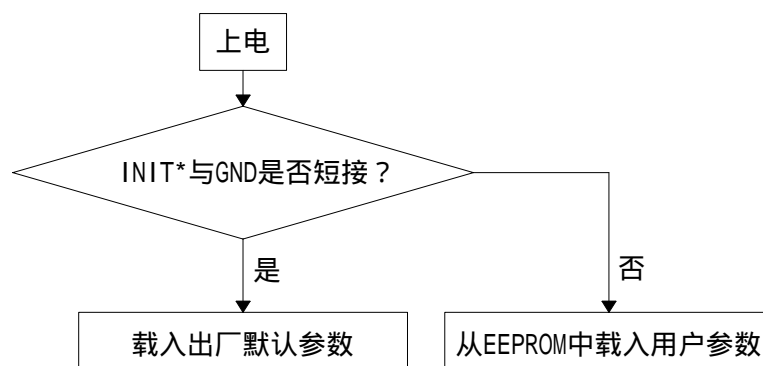
图2.5.2 IR-2190 启动过程及参数载入流程图
