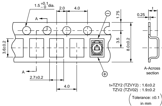
TZY2/TZV2系列
