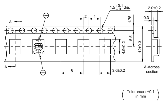
TZC3系列
