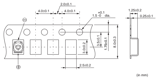
TZS2系列
