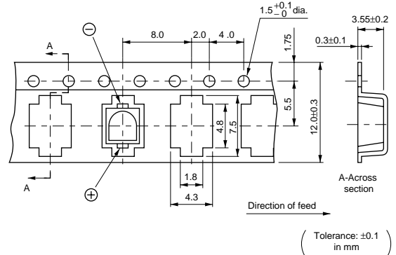
TZB4系列
