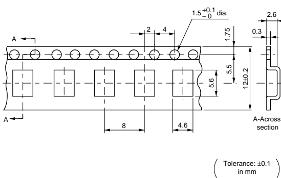
TZW4系列
