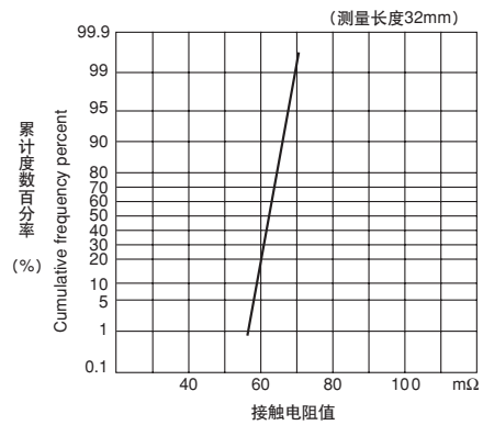
(2) 接触电阻值
