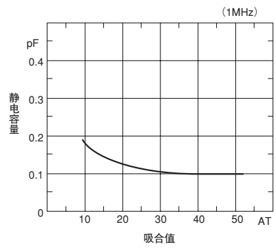
(5) 触点间静电容量
