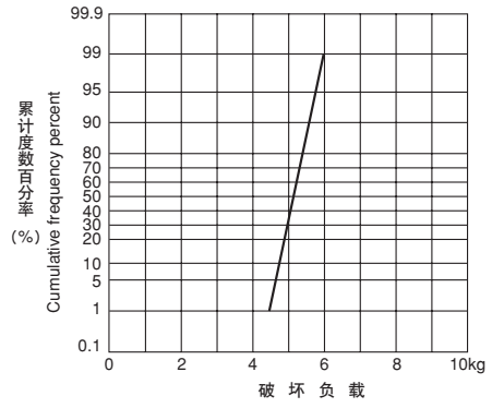
(2) 端子牵拉强度
