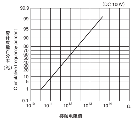
(4) 绝缘电阻值
