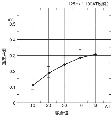
(1) 动作时间
