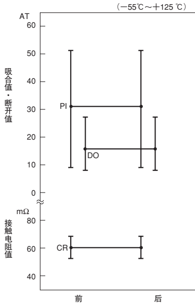
(4) 高温搁置
