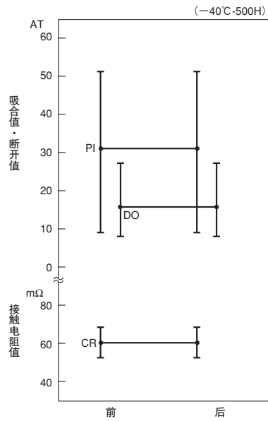
(5) 低温搁置
