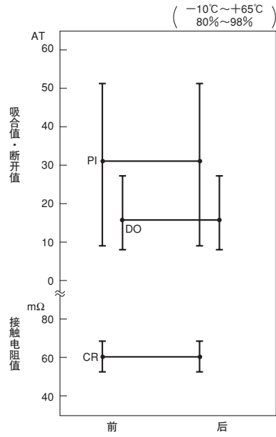
(3) 温湿度周期
