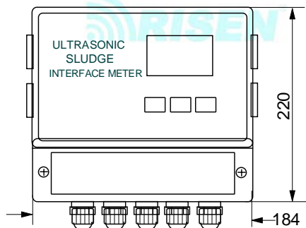
壁挂型仪表
