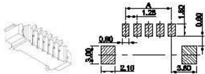
P.C.B LAYOUT
