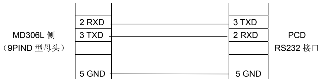
MD2-SAIA-RS232 连线图
