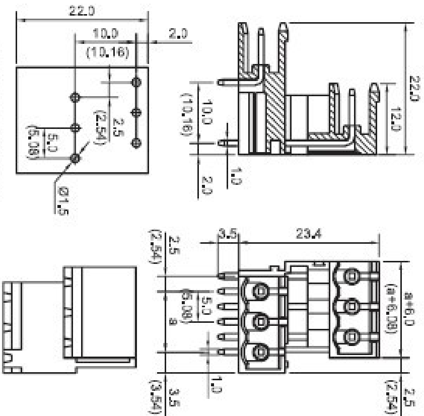
P.C.B LAYOUT
