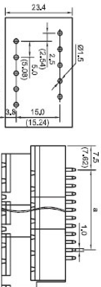
P.C.B LAYOUT
