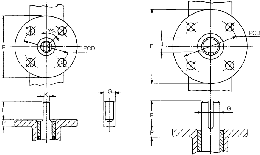
sizes 25-200 mm
