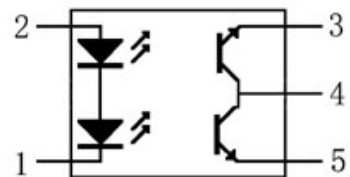
内部电路示意图
