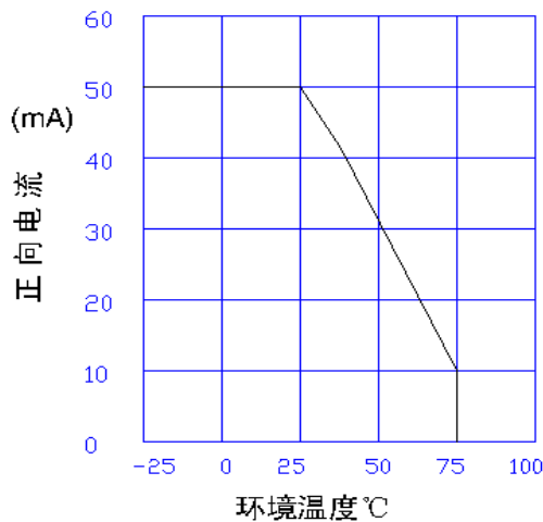
附图1. 正向电流与环境 温度曲线图
