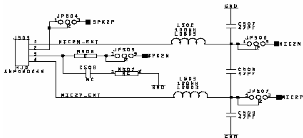
图 5-9 音频接口通道 2 电路参考设计原理图
