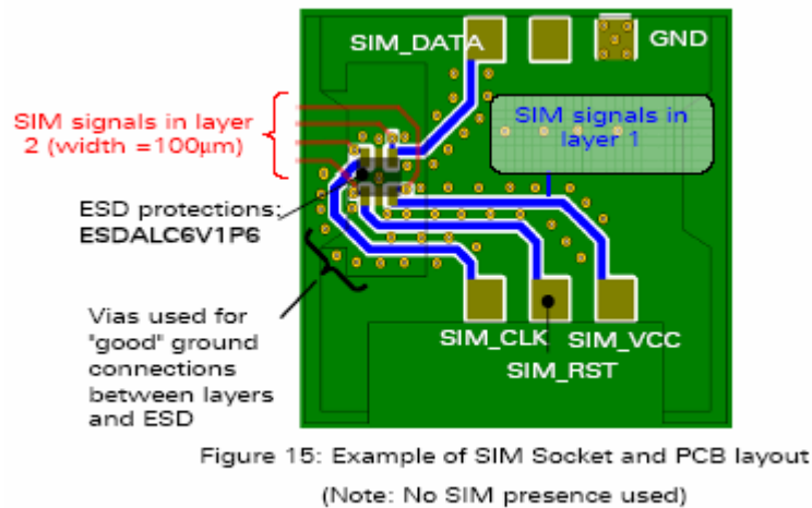
图 5-7 用户身份识别卡 SIM 电路参考设计 PCB 图
