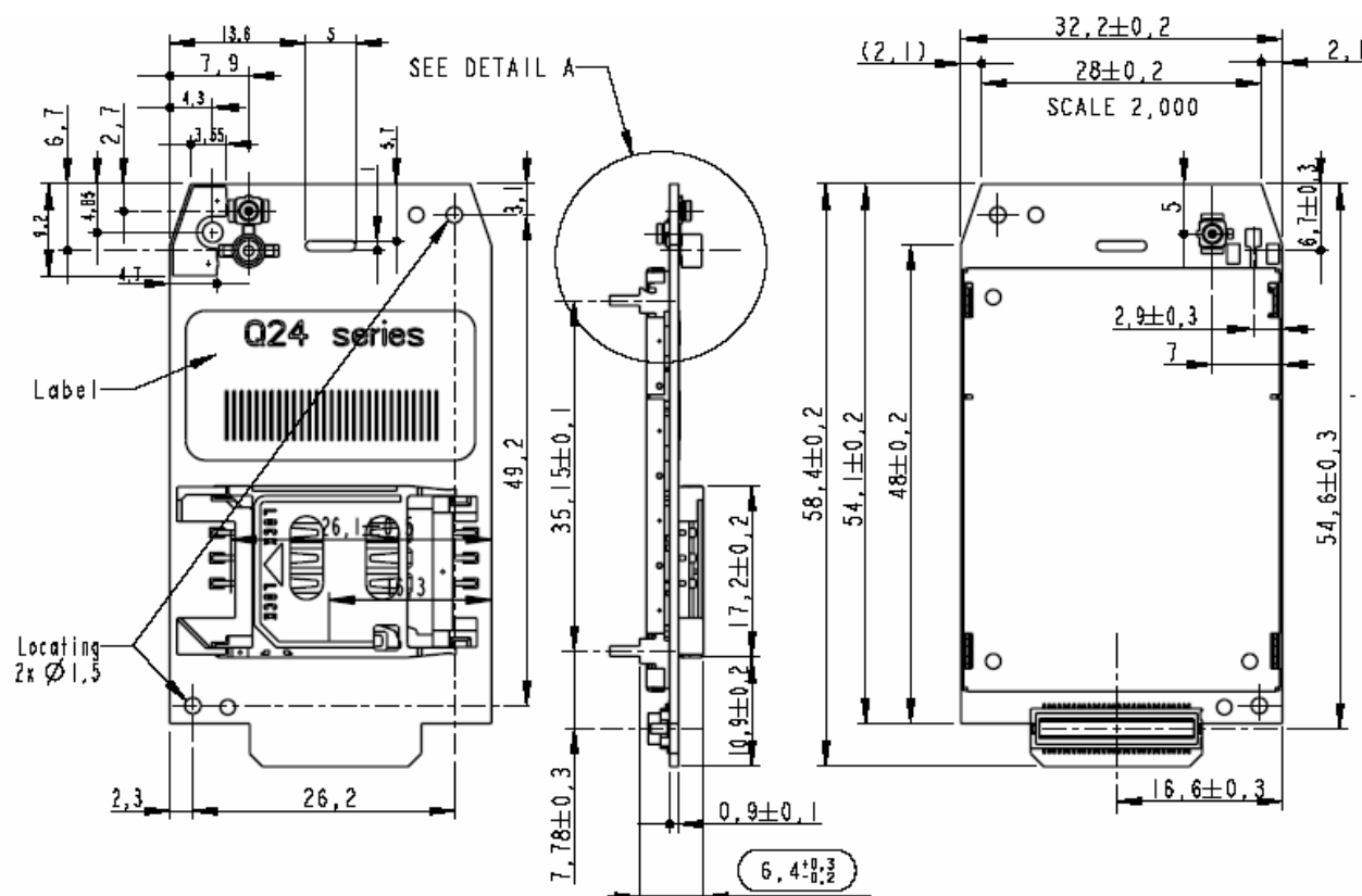
图 6-3 模块装配图 (底视图)
