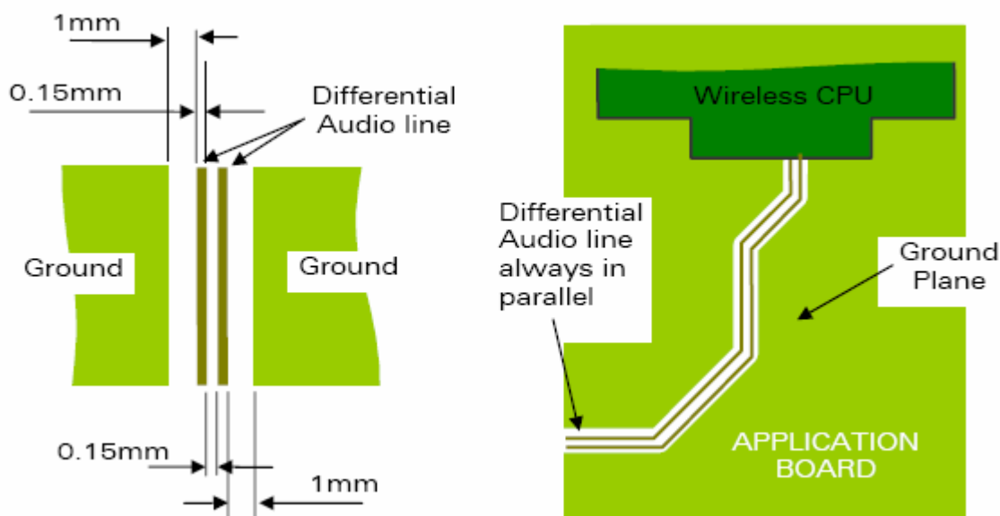
图 5—10 音频走线 PCB 参考
