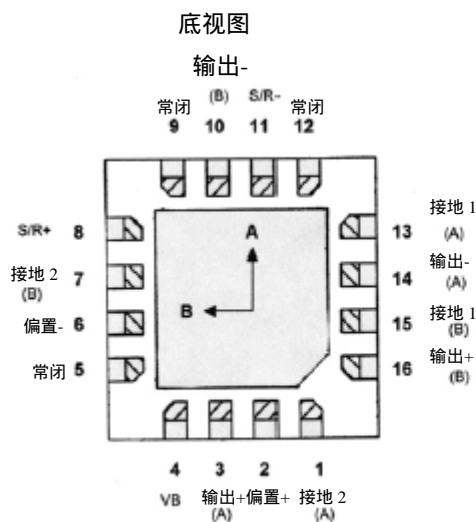
HMC1052L 引脚
