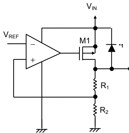
图17 电压稳压器电路
