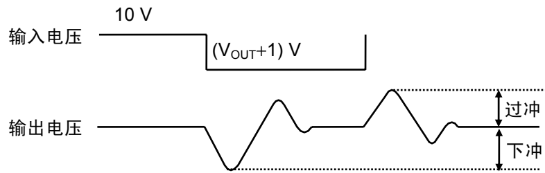
图 25 (V_{OUT}+1) V \leftrightarrow 10 V 的矩形波时(类型 1)
