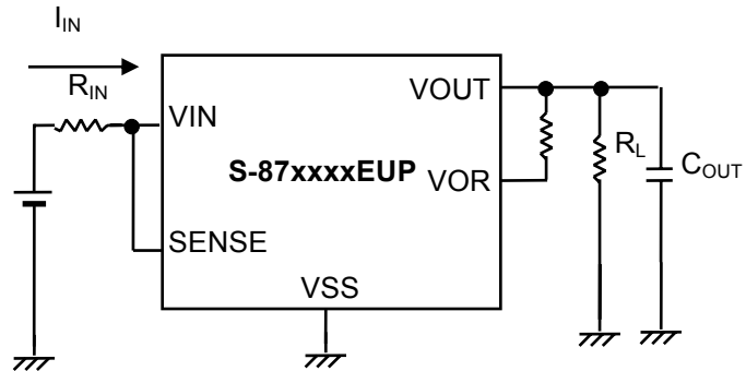
图 23 注意连接示例 2
