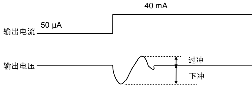
图 30 通过输出电流而引起输出电压的变动
