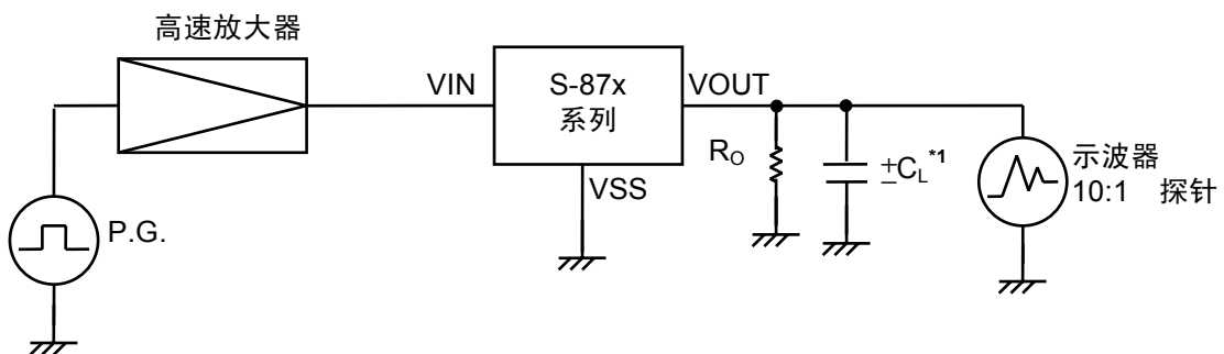
图 27 测定电路
