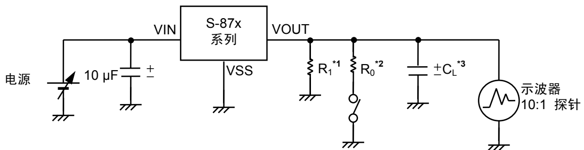
图 30 通过输出电流而引起输出电压的变动
