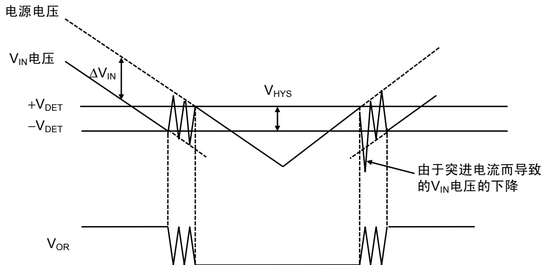
图 24 \Delta V_{IN} > V_{HYS} 时
