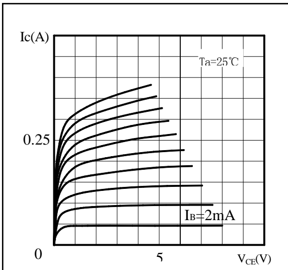
图3 输出特性曲线 ( I_C-V_{CE} )
