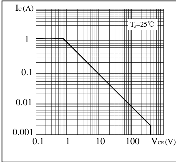
图1 安全工作区(直流)
