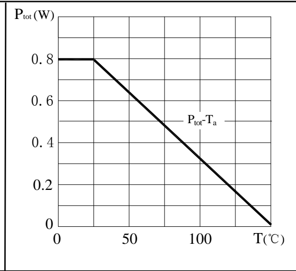
图2 P_{tot}-T 关系曲线
