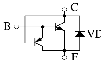
内部等效原理图
