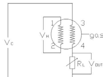
基本测试电路
