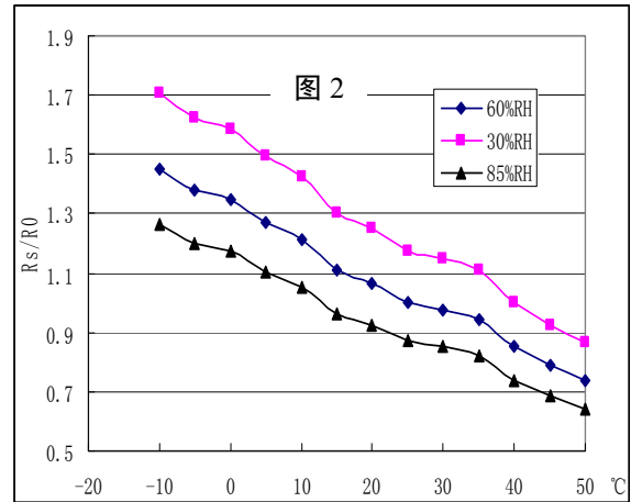
图2中 R_s 表示在含2000ppm丙烷、各种温/湿度下的电阻值； R_o 表示在含2000ppm丙烷、20°C/65%RH下的电阻值。
