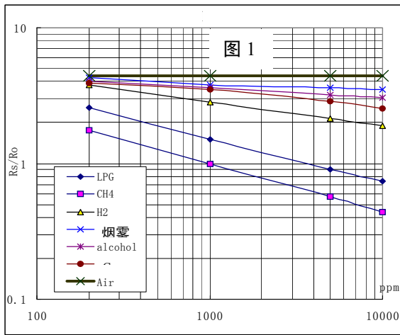
图1中 R_s 表示传感器在不同浓度气体中的电阻值； R_o 表示传感器在2000ppm丙烷中的电阻值。图中所有测试都是在标准试验条件下完成的。
