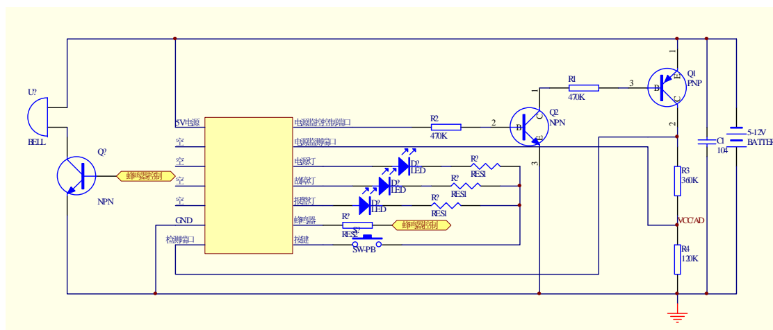
推荐应用原理图
