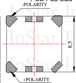
Unit:mm TOL: \pm 0.3
