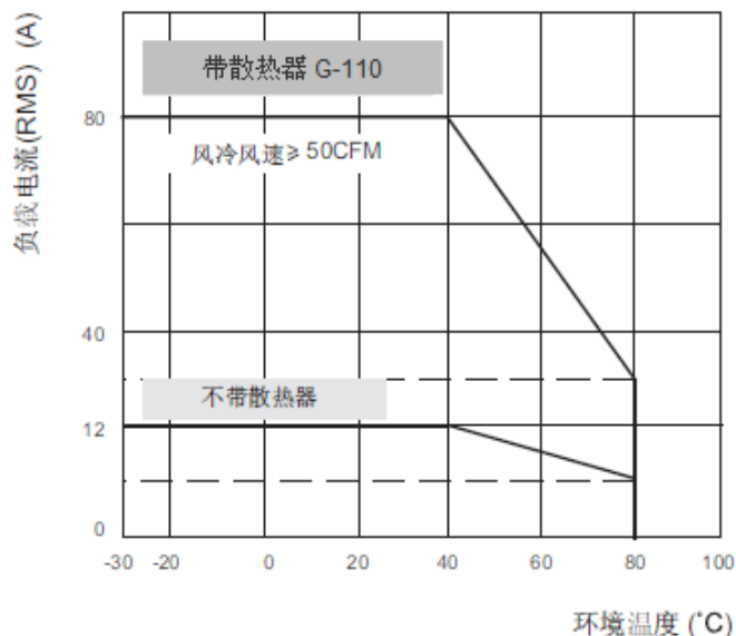
最大负载电流与环境温度曲线 (80A)
