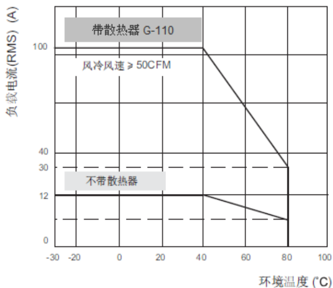
最大负载电流与环境温度曲线 (100A)
