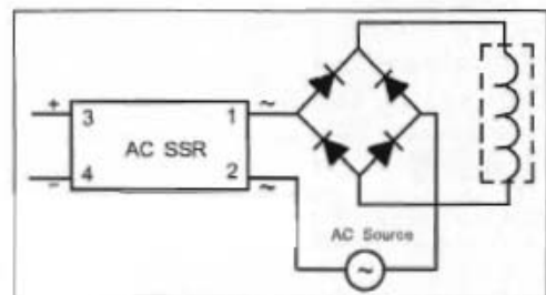
(6) 交流 SSR 驱动直流负载
