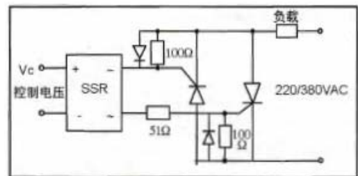
(4) 双单向硅功率扩展
