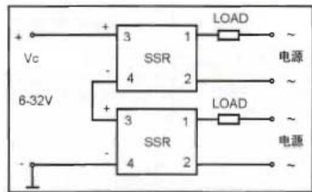
(1) SSR 的串联驱动
