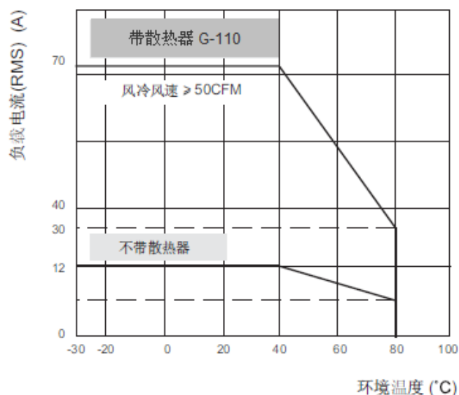
最大负载电流与环境温度曲线 (70A)
