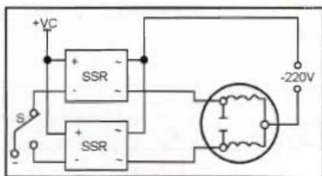
(5) 单向电机正反转
