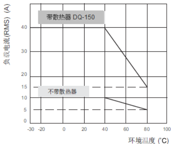
最大负载电流与环境温度曲线 (40A)
