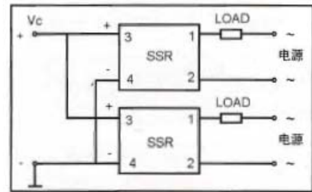
(2) SSR 的并联驱动
