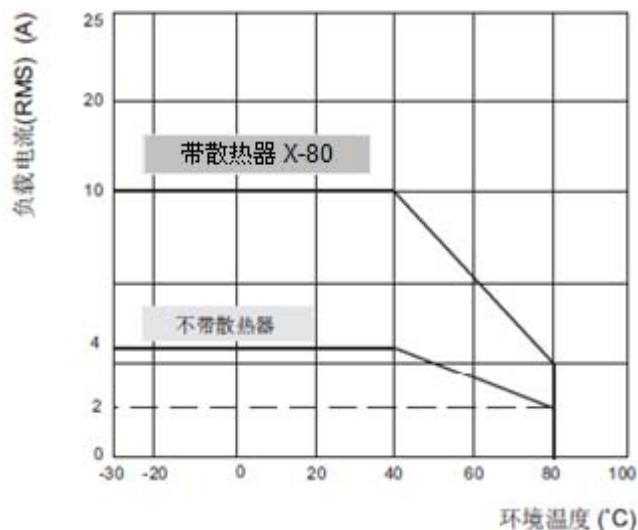
最大负载电流与环境温度曲线 (10A)
