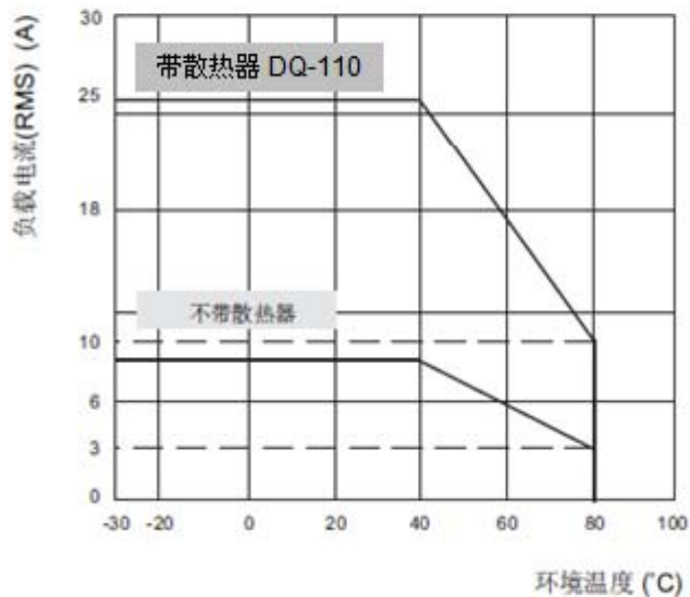
最大负载电流与环境温度曲线(25A)
