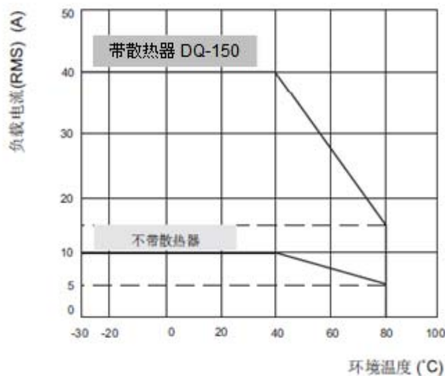
最大负载电流与环境温度曲线(40A)
