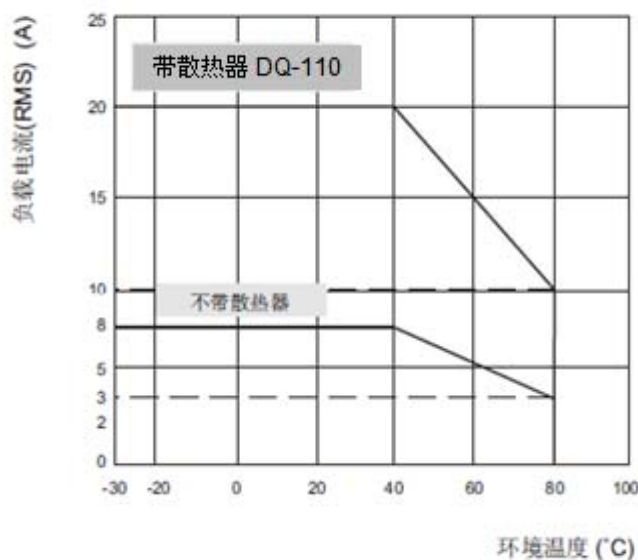
最大负载电流与环境温度曲线(20A)
