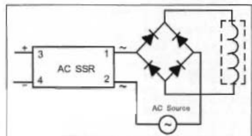
(6) 交流 SSR 驱动直流负载
