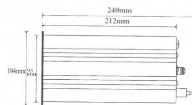
側視圖
