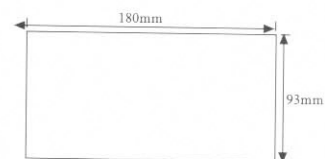
開孔圖
