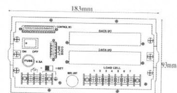
後視圖
