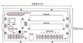
後視圖 Rear View
