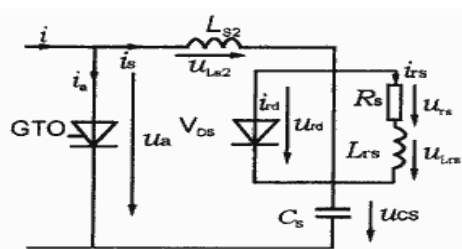
图 1 GTO 缓冲电路示意图
