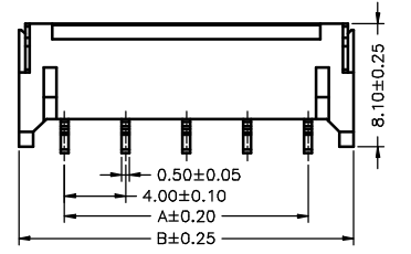
A4001WR-S-5P -GG
