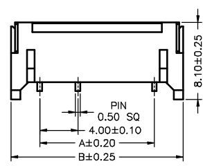
A4001WR-4P-137
