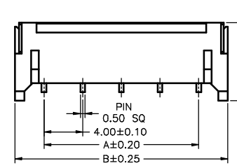
A4001WR-5P
