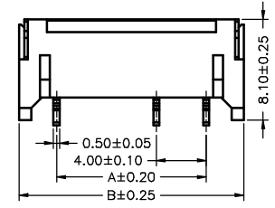
A4001WR-S-4P-157 -GG
