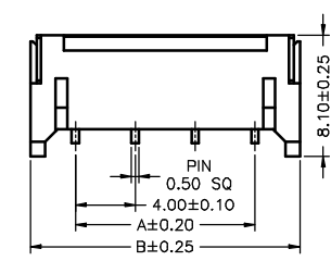
A4001WR-4P
