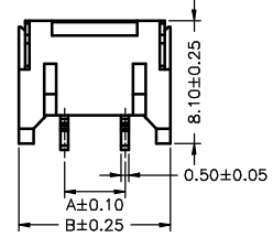
A4001WR-S-2P-1 -GG
