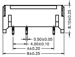
A4001WR-S-4P-137 -GG
