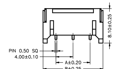
A4001WR-3P
