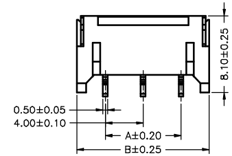
A4001WR-S-3P
