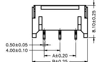
A4001WR-S-3P -GG
