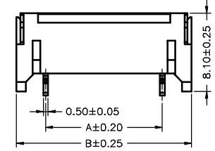
A4001WR-S-2P-3 -GG
