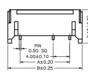
A4001WR-4P-157
