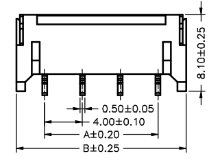
A4001WR-S-4P -GG
