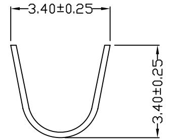
SEC:A-A
