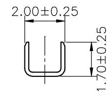
SEC:A-A
