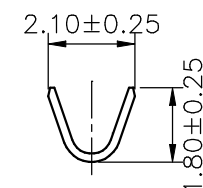
SEC:B-B
