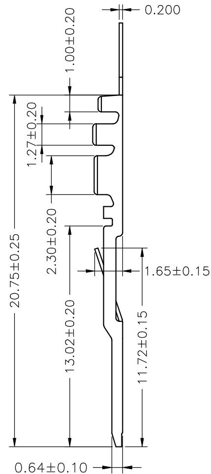
SEC:B-B
