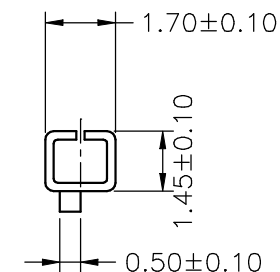
SEC:D-D
