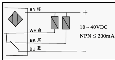
DC 三線式
