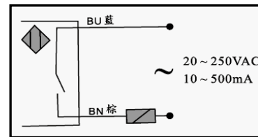
AC 二線式
