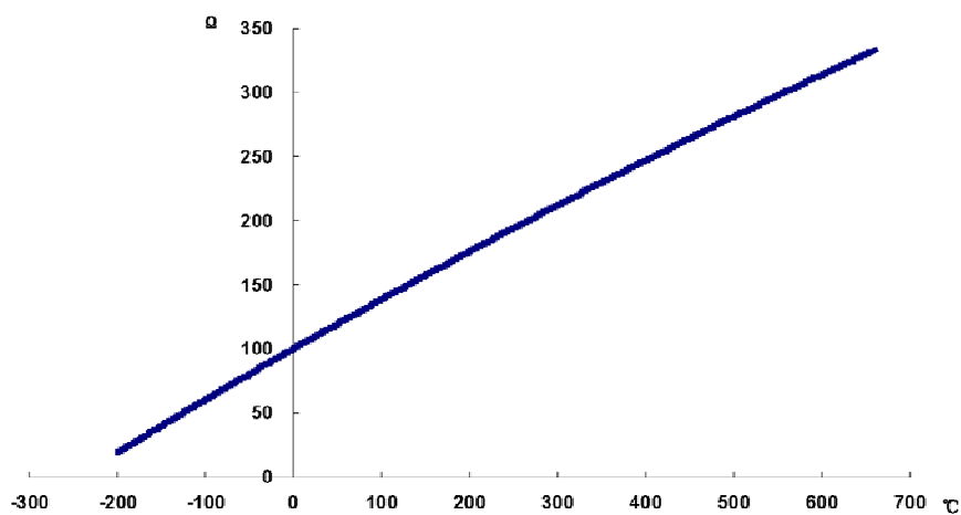
温度/阻值曲线表
