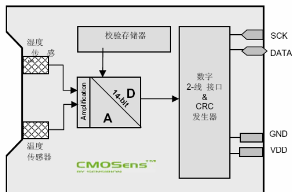
框图
