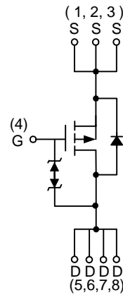
P-Channel MOSFET
