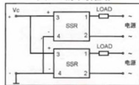
(2) SSR 的并联驱动
