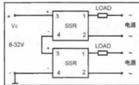
(1) SSR 的串联驱动
