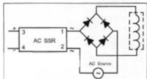
(6) 交流 SSR 驱动直流负载
