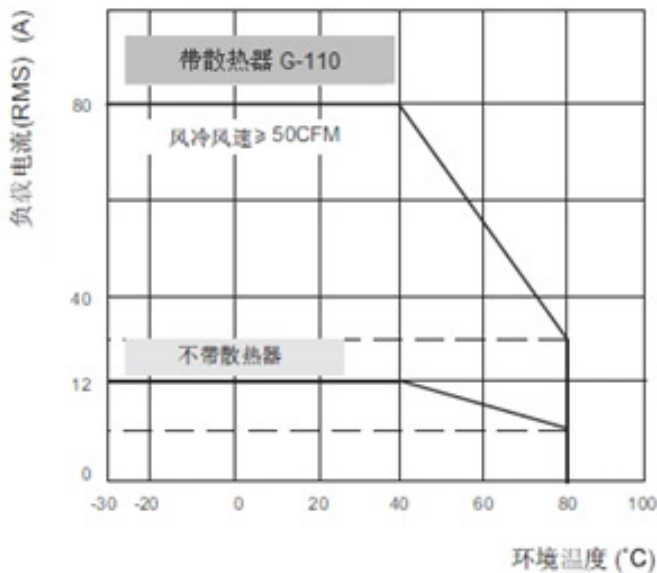
最大负载电流与环境温度曲线 (80A)
