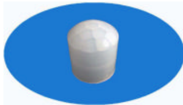
型号：8308-2(圆柱形) 焦距：9.5 角度：140° 距离：8m 尺寸：12.5 高度：14.30
