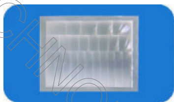
型号：7708-3 焦距：29.7 角度：79.8° 距离：10m 尺寸：45×58
