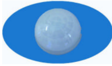
型号：8801-2 焦距：26 角度：100° 距离：5m 尺寸：55
