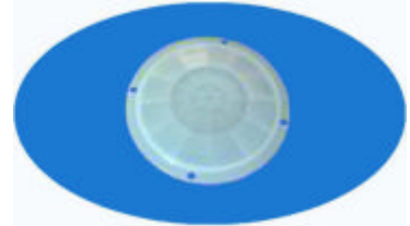
型号：8102-4 焦距：15 角度：120° 距离：7m 外径：43 内径：36
