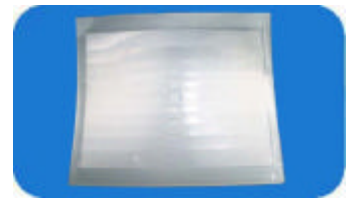
型号：7809(幕帘式透镜) 焦距：25 角度：90° 距离：12m 尺寸：49×57
