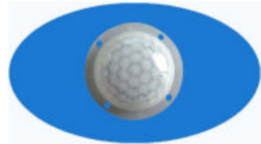
型号：8340 焦距：15 角度：120° 距离：10m 尺寸：外径 44.6 内径 35.00
