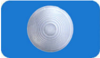
型号：8191(平板形) 焦距：26 角度：40° 距离比：8:1 尺寸：19
