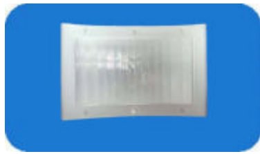
型号：RX-20 焦距：23 角度：120° 距离：8m 尺寸：24.5*38.2
