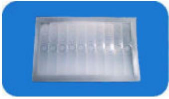
型号：8719(幕帘式透镜) 焦距：25 角度：90° 距离：10m 尺寸：34×53.5
