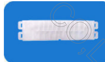
型号：7707-15 焦距：25 角度：120° 距离：12m 尺寸：82.5*20
