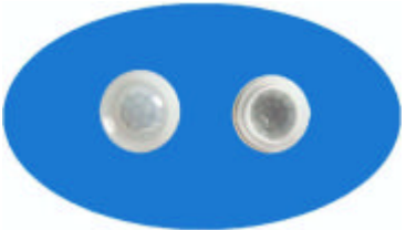
型号：7709-3 焦距：9.0 角度：120° 距离：8m 尺寸：外径 17.8 内径 12
