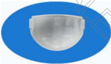
型号：RX-40 焦距：20 角度：120° 距离：8m 尺寸：55 1/4圆
