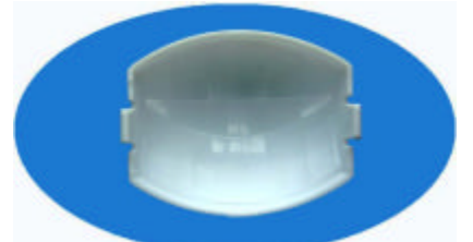
型号：RX-50 焦距：25 角度：120° 距离：10m 尺寸：高:55 宽:60 sales@salens.cn
