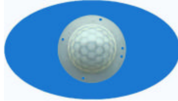
型号：8320 焦距：17.5 角度：120° 距离：9m 尺寸：外径 44.8 内径 32.00
