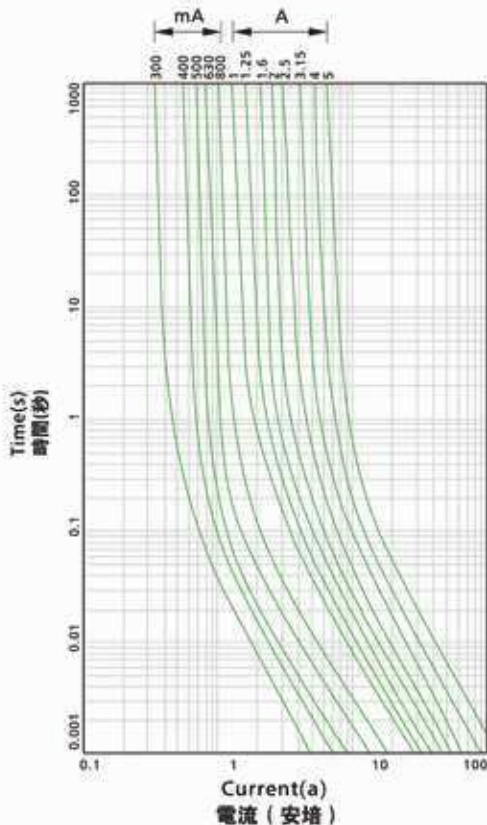
Time-Current Characteristics 電流-時間曲線圖
