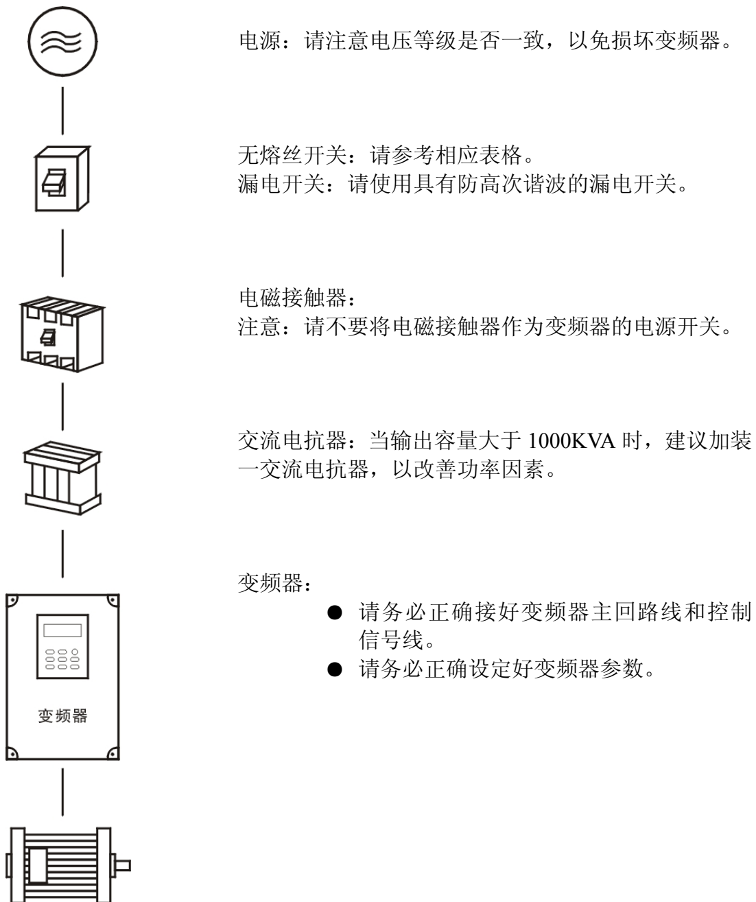
(1)主回路配线示意图
