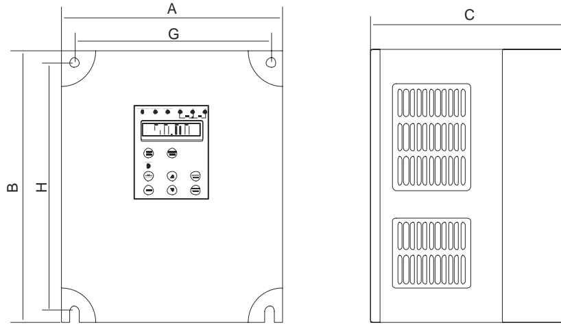
附录二、外形及安装尺寸
