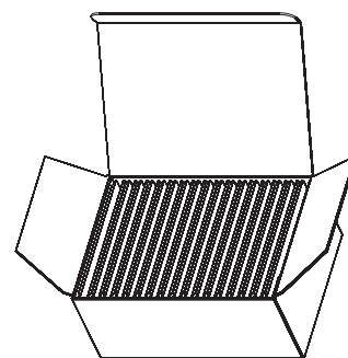
box size(L210*W150*H92MM)
